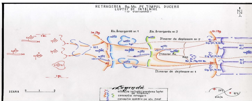
Figura 3. Exemplu de desfășurare a retragerii de către brigada mecanizată când structurile participante folosesc metoda întârzierii din poziții succesive (sursa: Irinel
