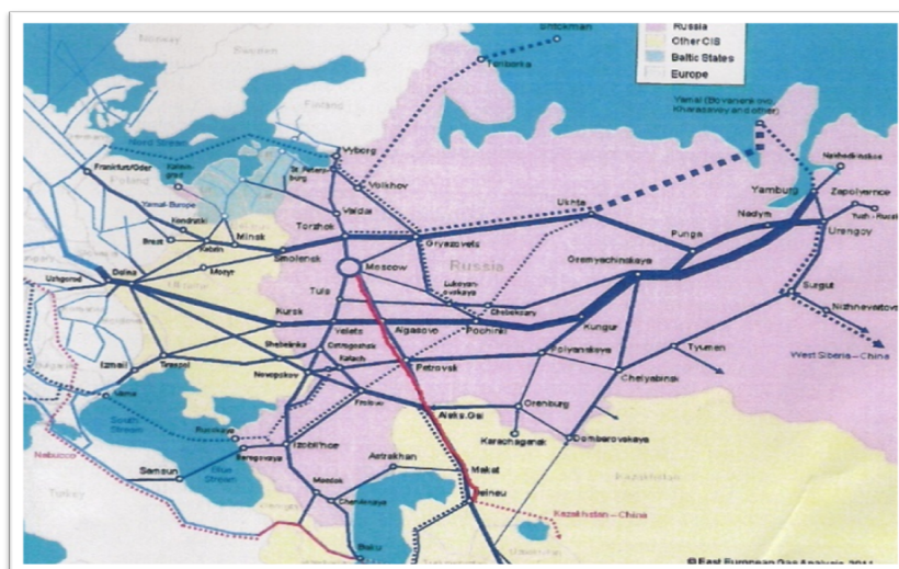
Figura nr. 3. Structura rețelei conductelor de gaze a URSS Sursa: East European gas Analysis 4
