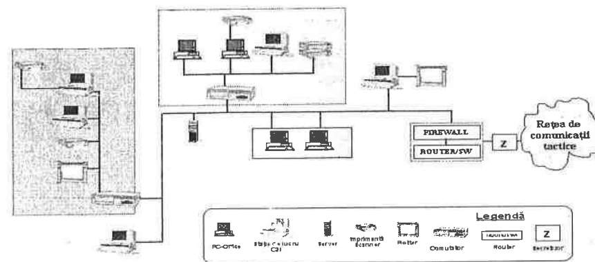
Figura 3 Structura unei rețele locale de calculatoare
